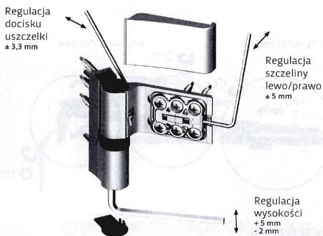
Rys. 16 Zawias drzwi zewnętrznych
