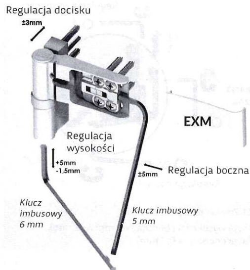
Rys. 17 Zawias drzwi wewnętrznych oraz drzwi tarasowych otwieranych na zewnątrz
