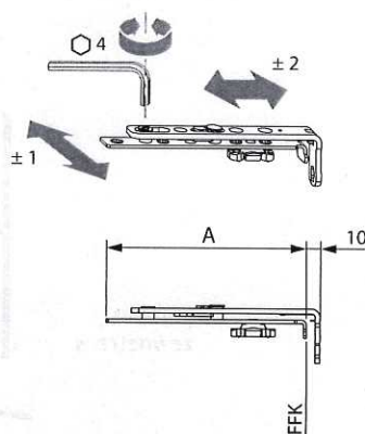
Rys. 10 Rozwórka R
