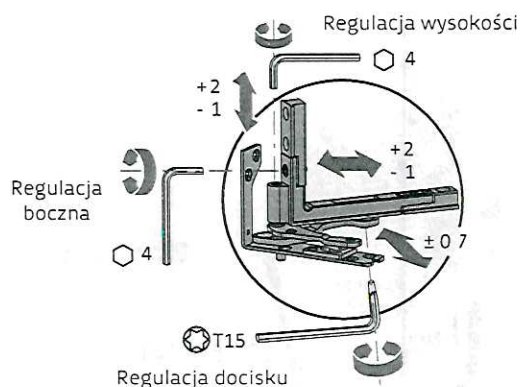
Rys. 11 Zawias dolny
