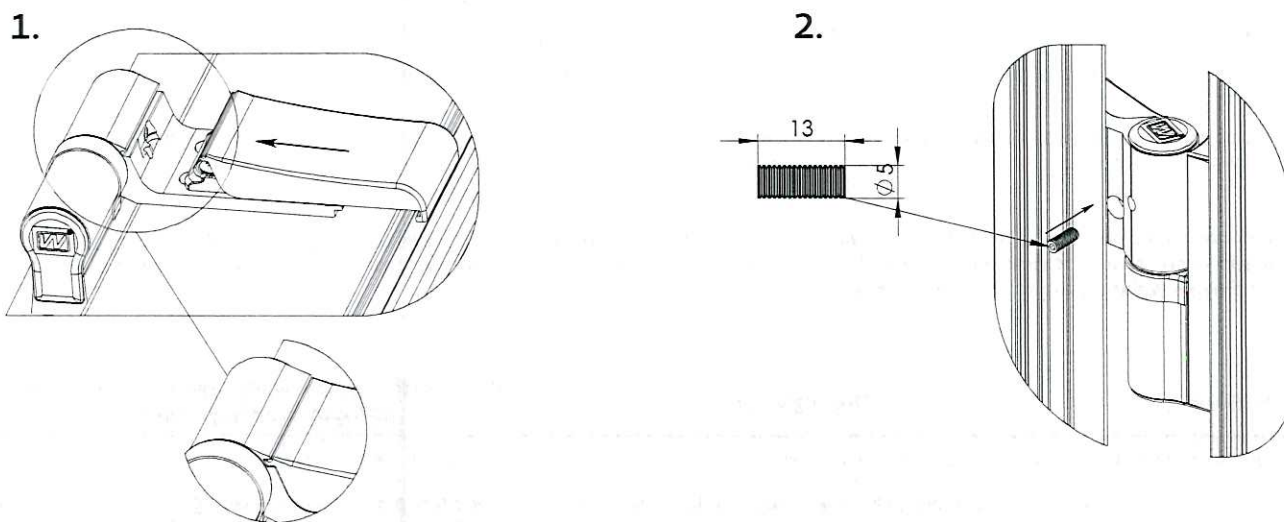
Rys. 18 Zabezpieczenie płytki za pomocą wkręta przy otwartych drzwiach Należy użyć klucza imbusowego 2,5 mm
