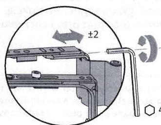
Regulacja boczna
