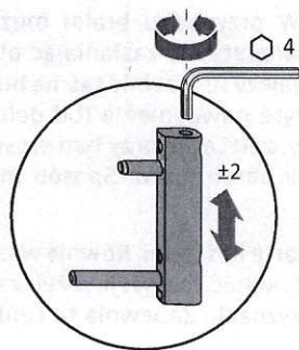
Rys. 7 Zawias skrzydła
