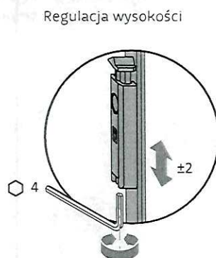
Rys. 13 Zatrask balkonowy komfort.
