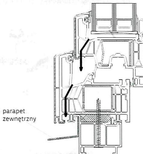
Rys. 6 Schemat montażu parapetu zewnętrznego przy krytym odwodnieniu
