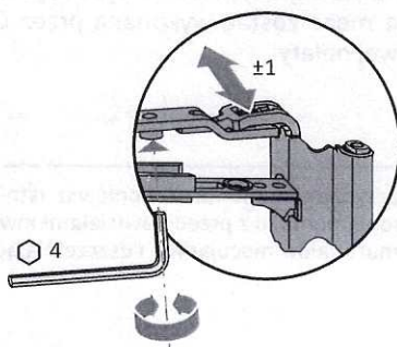
Rys. 9 Rozwórku RU
