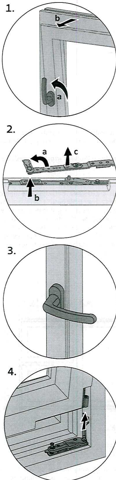
Rys. 2 Zakładanie i zdejmowanie skrzydła
