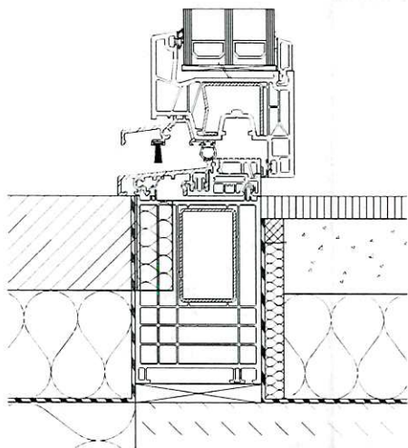
Rys. 5 Schemat montażu niskiego progu
