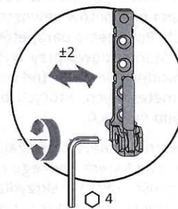
Rys. 8 zawias ramowy
